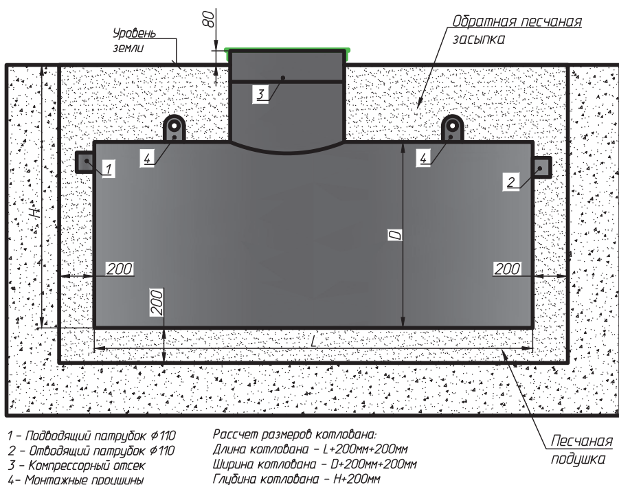
Монтажная схема станций KANN серии ECO
